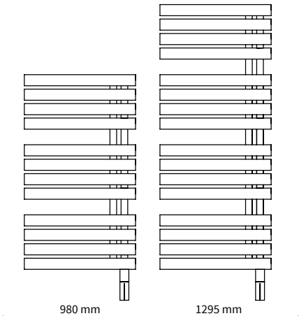
UKŁAD SUSZARKI PRZY WYSOKOŚCI: electric towel rail shape and design with the height:
